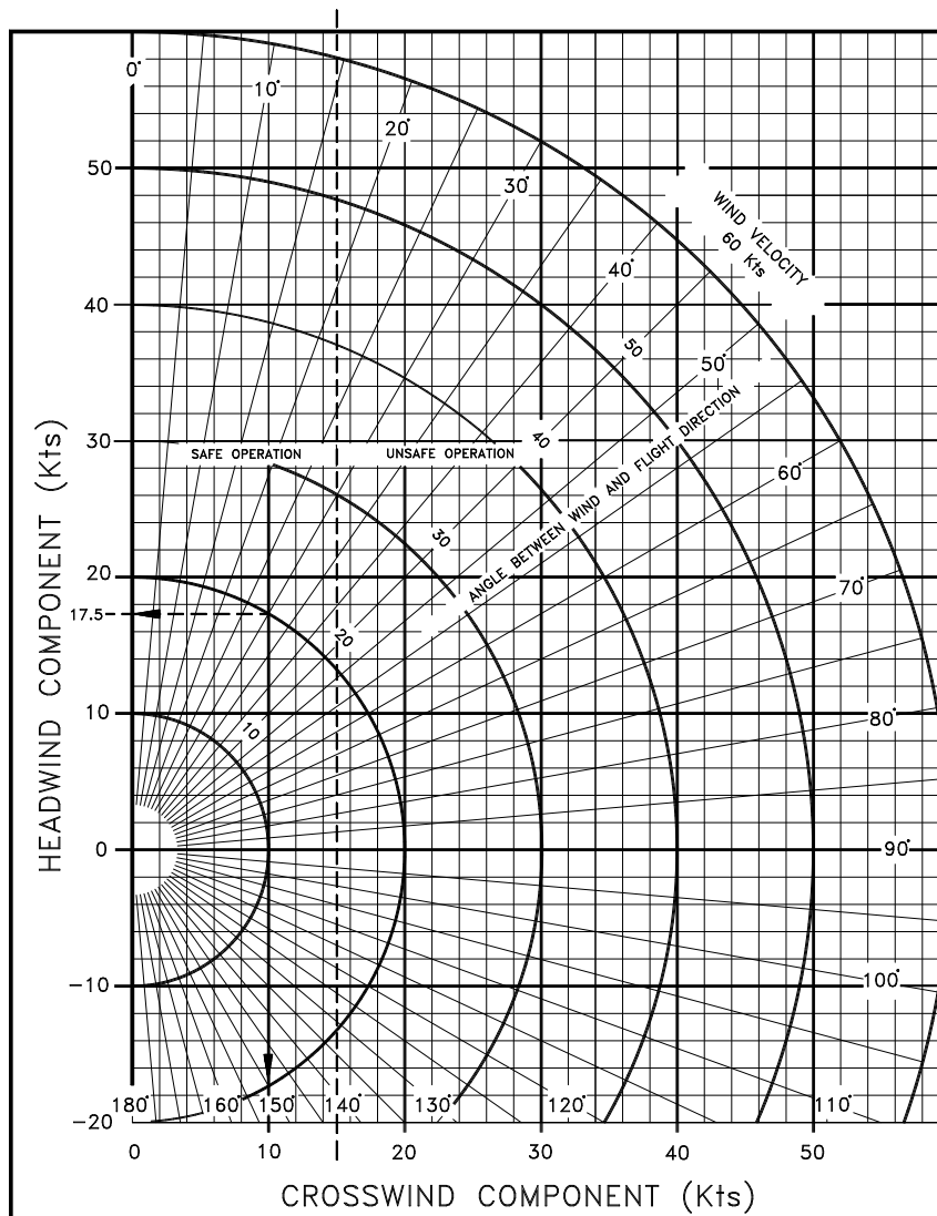
FIG. 5-2. CROSSWIND CHART
